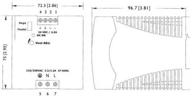
DPP100-24 Dimensions
